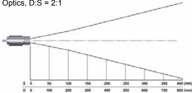
Optics, D:S = 2:1
